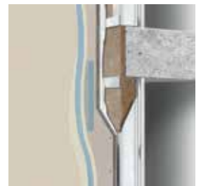
جزئیات اجرای دیوار خارجی با پوشش نمای رنگ آمیزی
