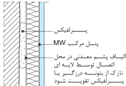
اتصال پوشش کاری به دیوار زمینه
