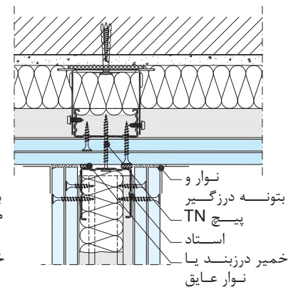
اتصال دیوار جداکننده به دیوار پوششی
