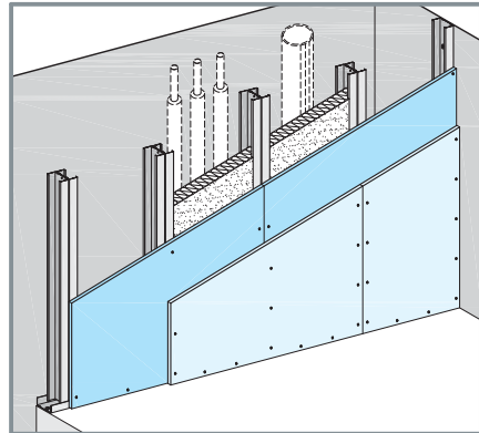
دیوار پوششی W629 (F30 : پوشش کاری ۱۲/۵×۲ م.م)
