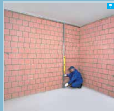
۴ انتقال تصویر رانر سقف به کف (با استفاده از استاد و تراز)
