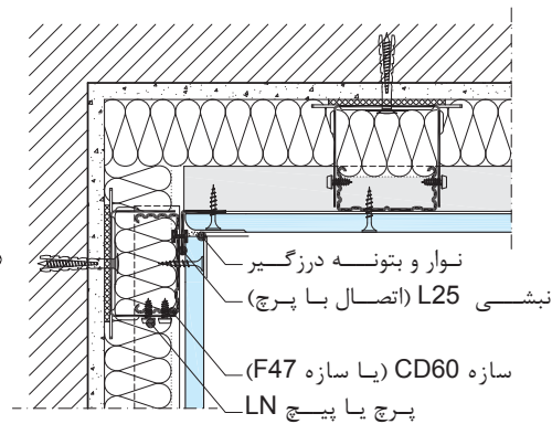
اتصال گوشه داخلی
