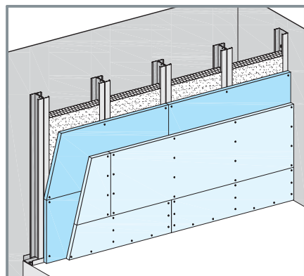
دیوار پوششی W629 (F90 : پوشش کاری ۲۰×۲۰ یا ۲۵×۲ م.م)
