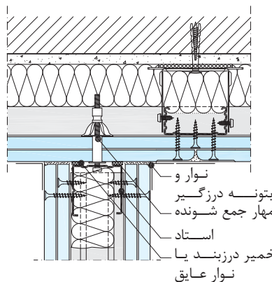
اتصال دیوار جداکننده به دیوار پوششی
