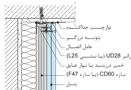
اتصال به سقف
