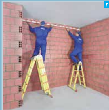
استقرار کرم بالا
