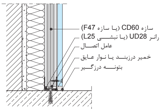
اتصال به کف
