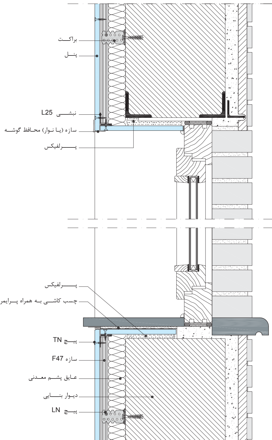
پوشش کاری دور پنجره و جزئیات نصب سنگ کف پنجره
