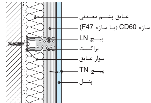
اتصال به دیوار زمینه
