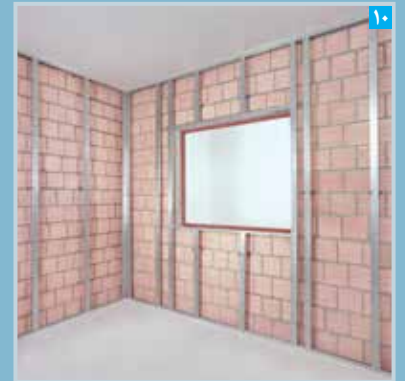
۱۰ زیرسازی و قاب بندی بازشوی پنجره تکمیل شده
