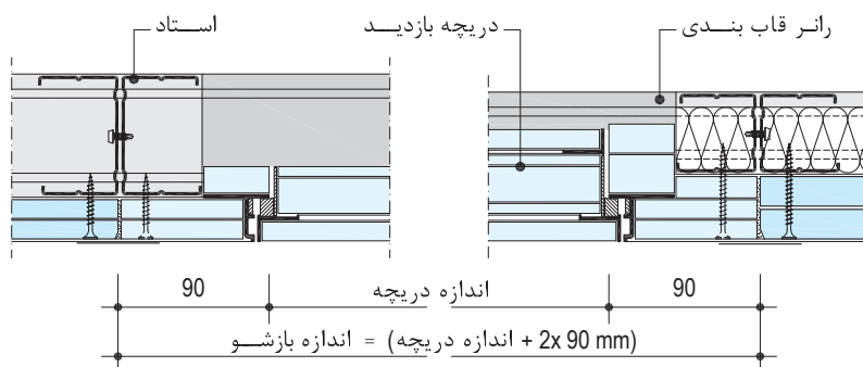
جزئیات نصب دریچه بازدید (F30)
