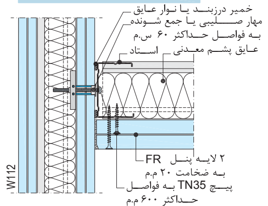
اتصال به دیوار خشک جانبی (F90)
